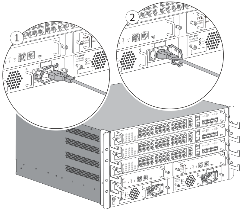
图3-2 连接电源线示意图
