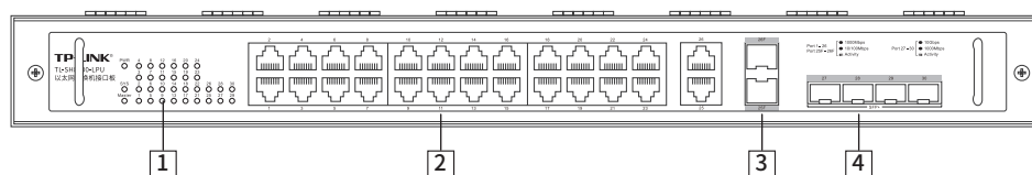
图1-11 TL-SH8430-LPU结构示意图
