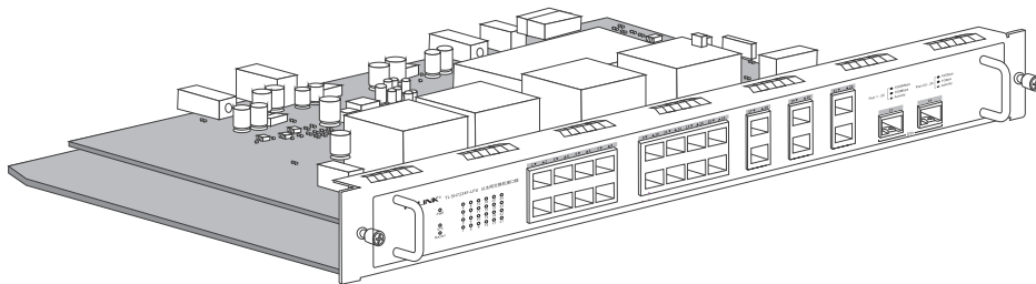
图1-12 TL-SH7224F-LPU业务板外观
