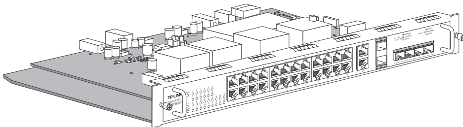
图1-10 TL-SH8430-LPU业务板外观
