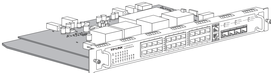
图1-14 TL-SH8430F-LPU业务板外观
