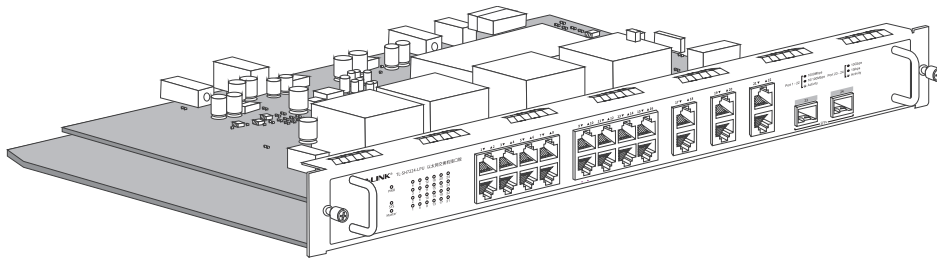
图1-8 TL-SH7224-LPU业务板外观
