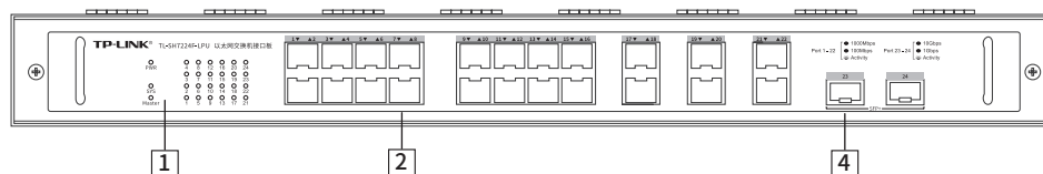
图1-13 TL-SH7224F-LPU结构示意图
